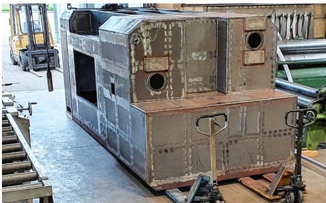
Eine Stahlkonstruktion für eine Bahnbaumaschine.
